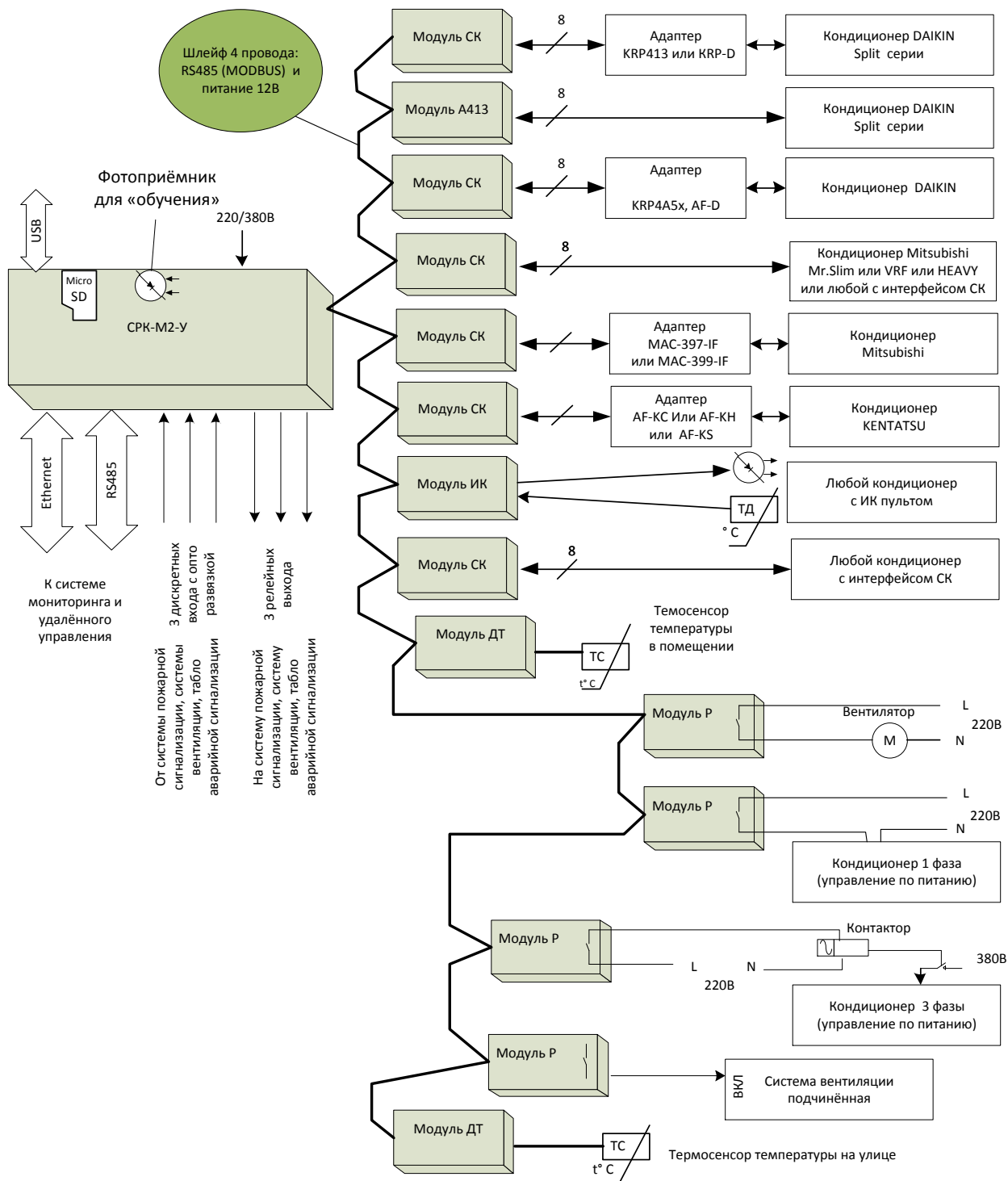
Рисунок 1 – Структурная схема системы на базе СРК-М2
